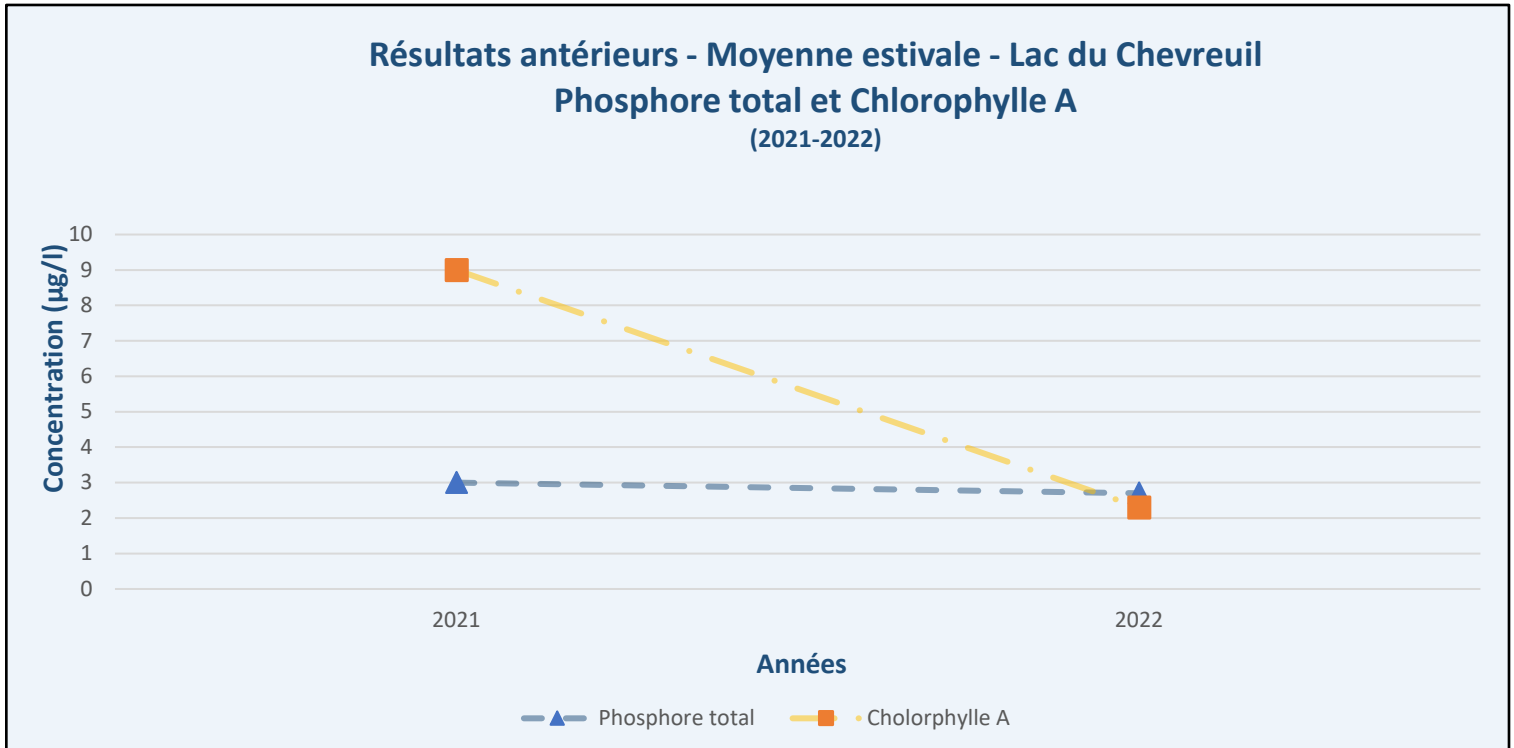
Figure 9 - Résultats antérieurs – Phosphore total – Chlorophylle A – Lac du Chevreuil (CH1)
