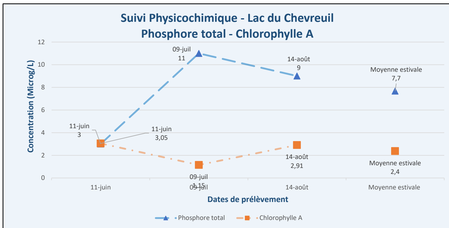
Figure 6 - Résultats – Suivi physicochimique 2022 (PT,Chla) – Lac du Chevreuil (CH1)
