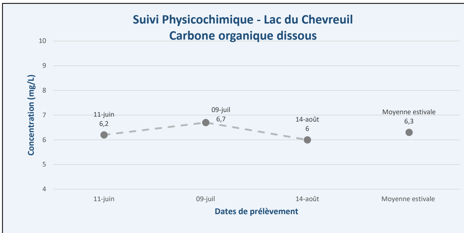
Figure 7 - Résultats – Suivi physicochimique 2022 (COD) - Lac du Chevreuil (CH1)
