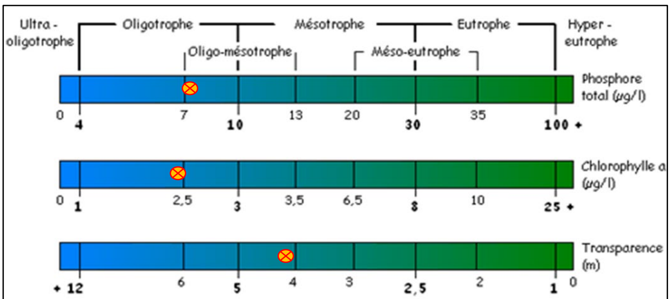
Figure 8 - État trophique 2022 - Station 1 - Lac du Chevreuil (CH1)
