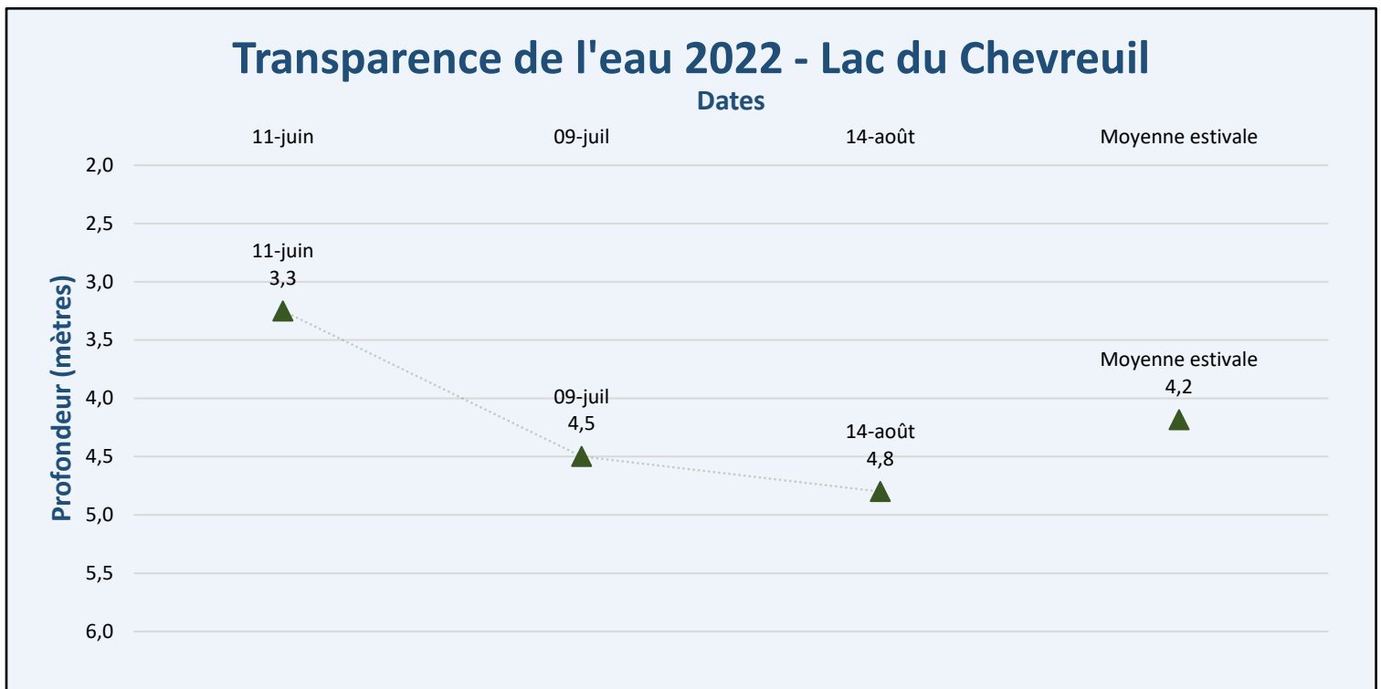
Figure 5 – Résultats - Transparence de l'eau 2022 - Lac du Chevreuil
